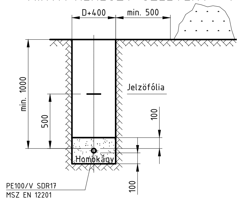
MINTA KERESZT-SZELVÉNY M 1:20
